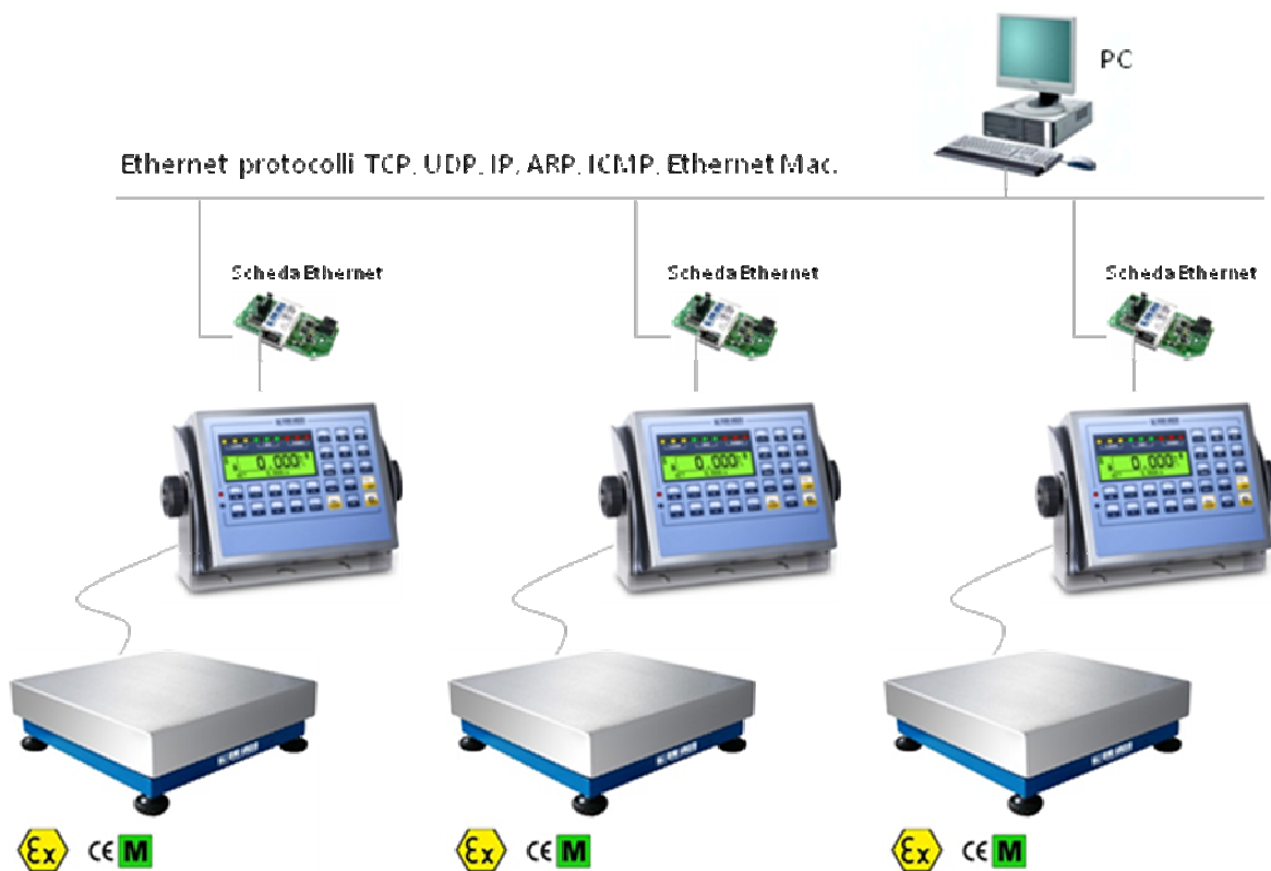
Fig. 4 Es. Rete aziendale con bilance controllo peso +/- CPWS-BVB
