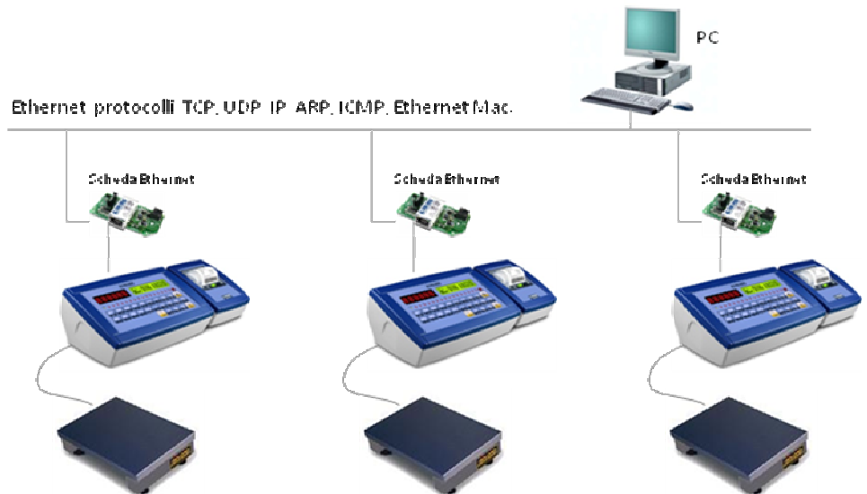
Fig. 2 Es. Rete aziendale con bilance KDQ-BVB
